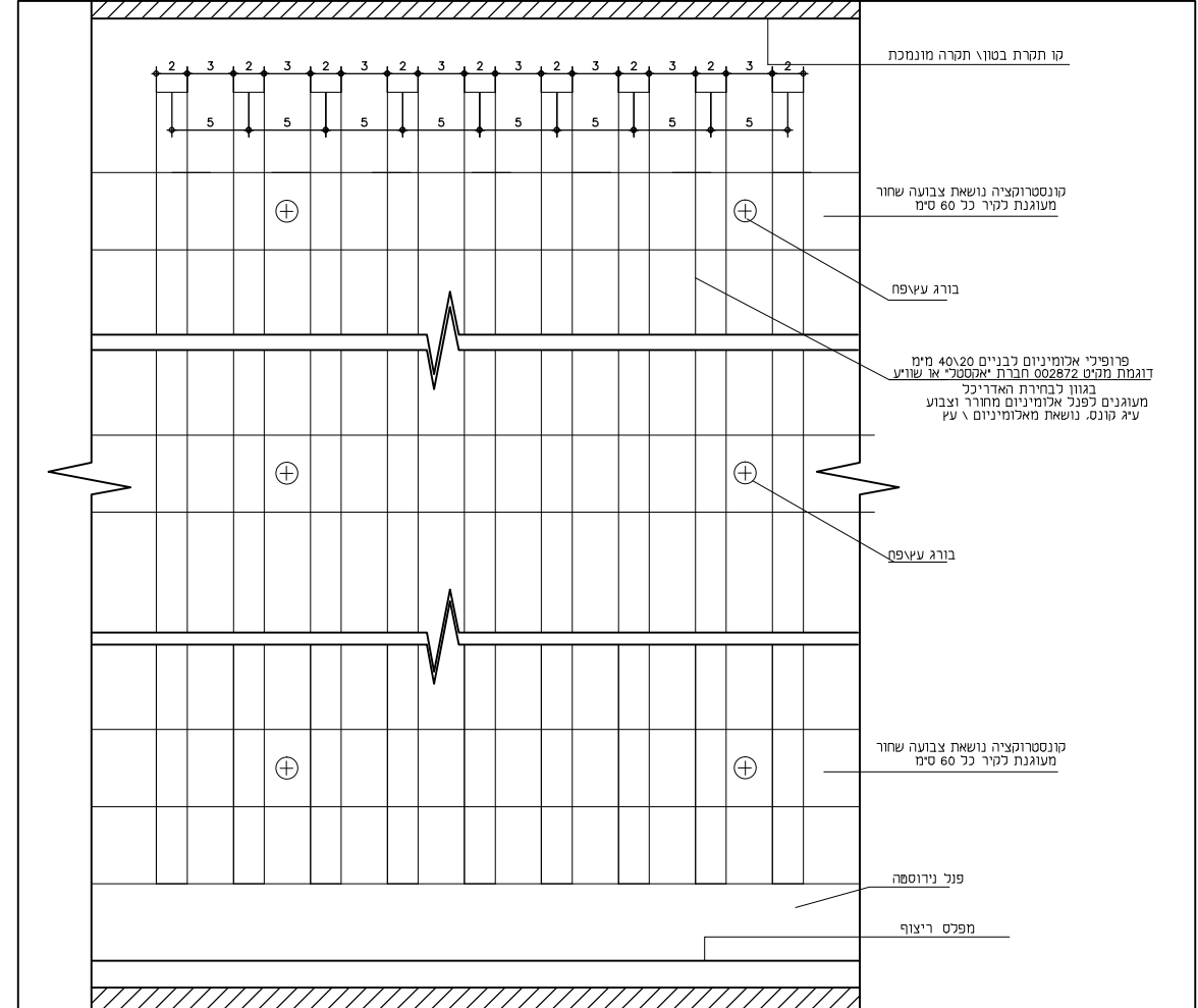
פרט חזית
