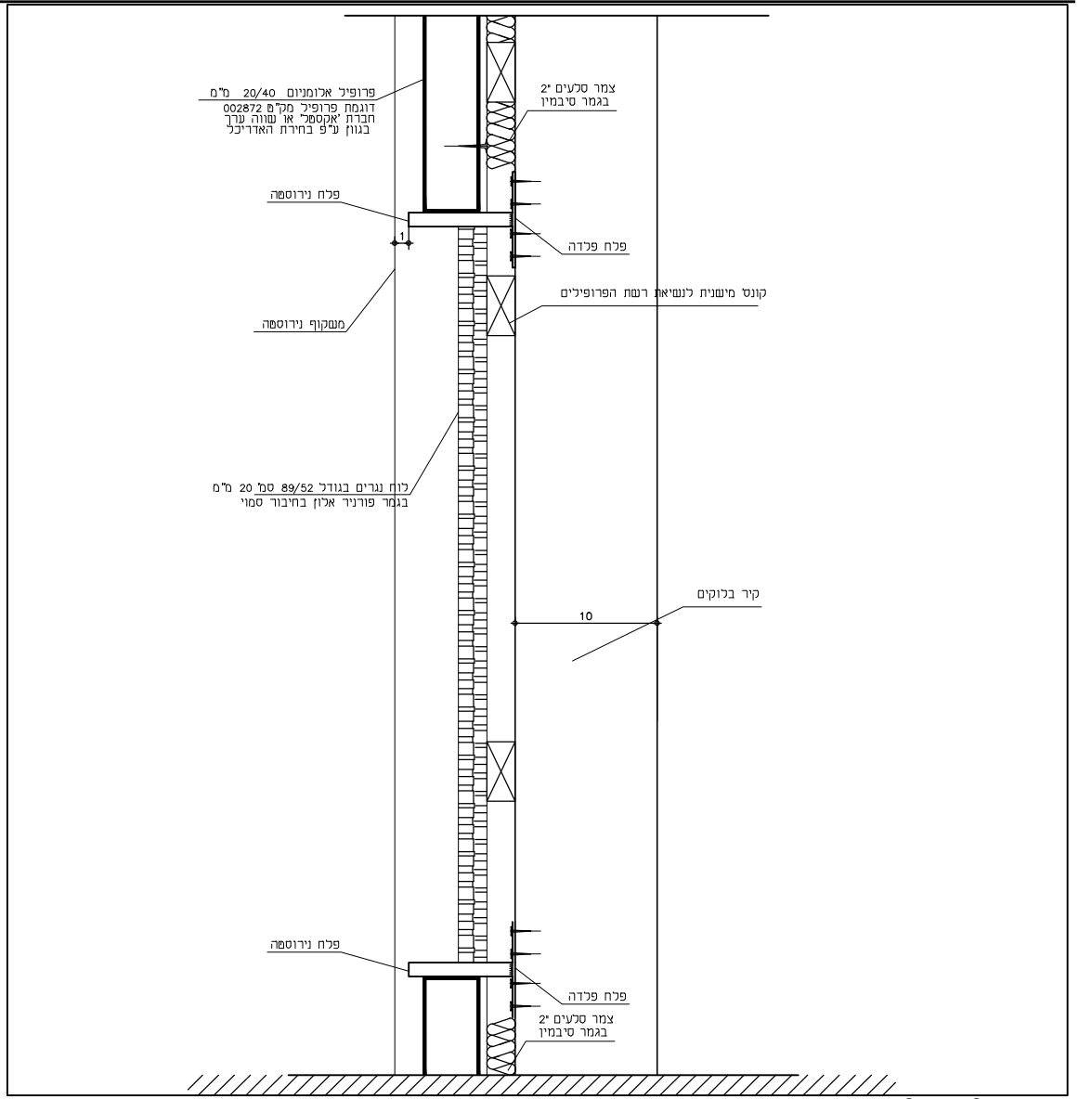
חתך 2-2
