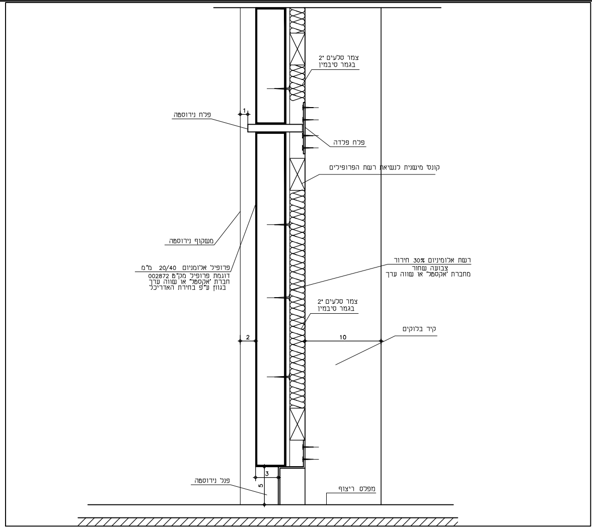
חתך 3-3
